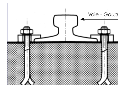
2 Montage sur béton Rail installation on concrete
